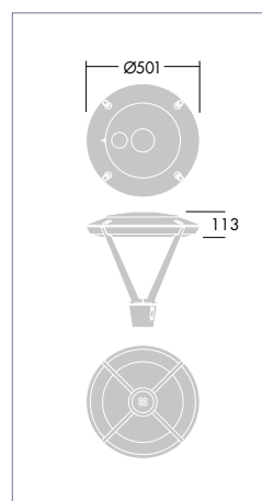
Montage porté avec manchon Ø 76 mm
