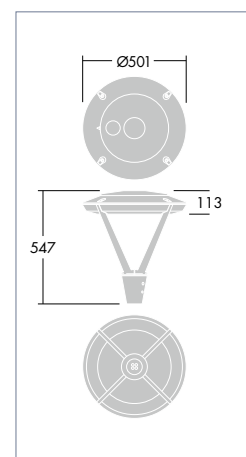
Montage porté avec manchon Ø 60 mm
