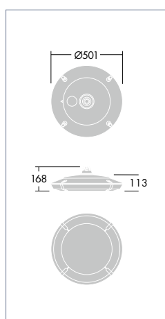
Montage suspendu
